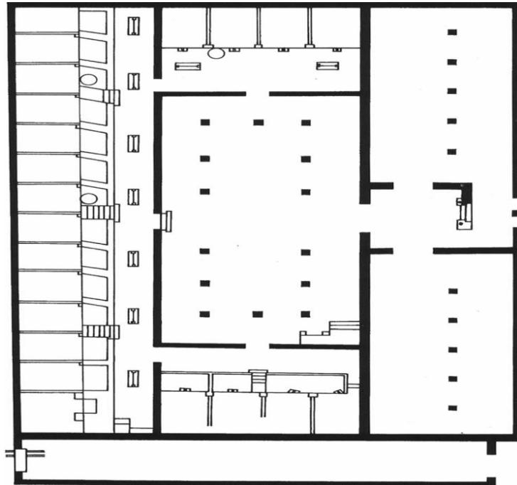
الشكل رقم 08 يمثل: مخطط تقريبي لمعصرة خربة أعقوب المرجع: Camps (H.F), Huile, op-cit, p 5.
